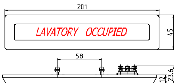
Sign «Lavatory Occupied» P/N 336303.003
