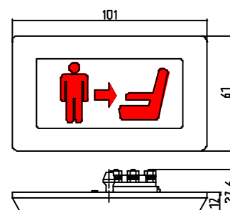
Sign «Return To Seat» P/N 336303.004
