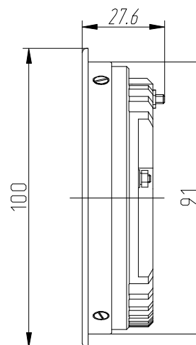
Габаритные размеры, мм
