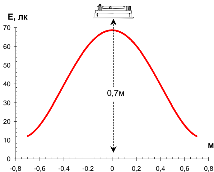
Распределение освещенности E
