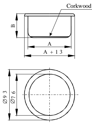
Подстаканник ИАРС.325881.002
