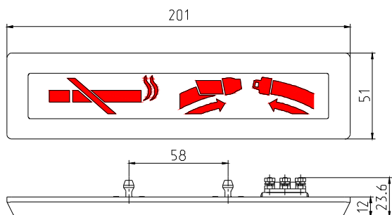
Табло КР-1 «Не курить. Пристегнуть ремни» ИАРС.336303.001
