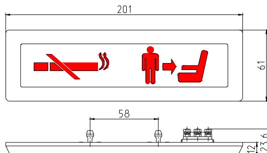
Табло КМ-1 «Не курить. Вернитесь на место» ИАРС.336303.002
