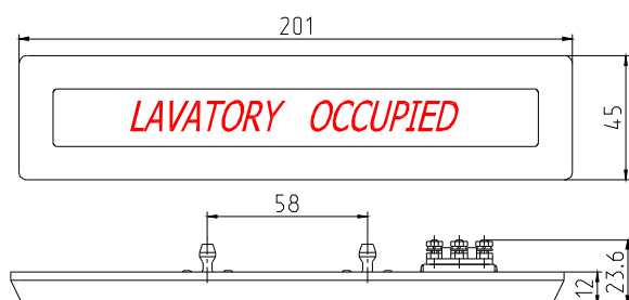
Табло ЗТ-1 «Туалет занят» ИАРС.336303.003
